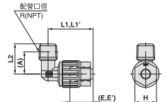
公牙L型彎頭：LQ3L-M
