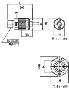
公牙L型彎頭：LQ2L-M
