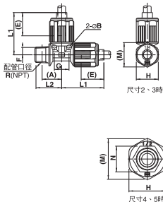
公牙3通接頭：LQ2R-M
