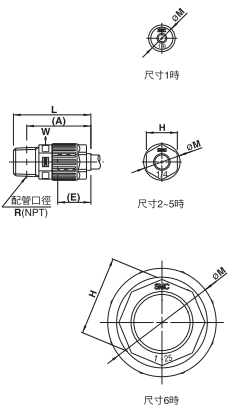
公牙接頭：LQ1L-M
