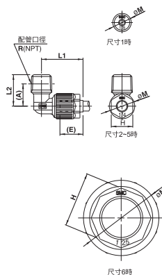
公牙L型彎頭：LQ1L-M
