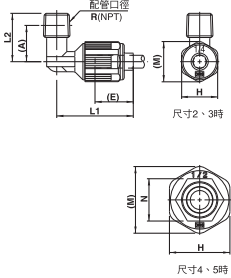
公牙L型彎頭：LQ2L-M
