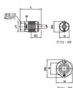
母牙L型彎頭：LQ2L-F
