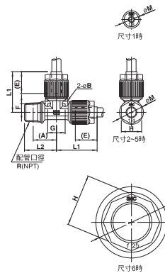
公牙3通接頭：LQ1R-M
