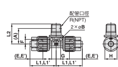
公牙分流接頭：LQ3B-M
