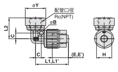
母牙L型彎頭：LQ3L-F
