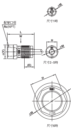
母牙L型接頭：LQ1L-F
