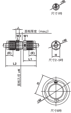
公牙接頭：LQ2H-M
