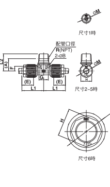
公牙分流接頭：LQ1B-M
