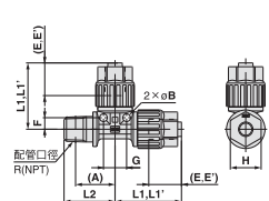
公牙3通接頭：LQ3R-M
