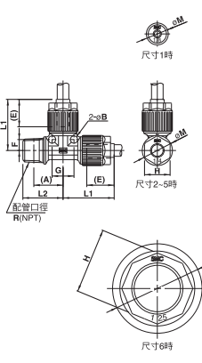
公牙分流接頭：LQ1B-M
