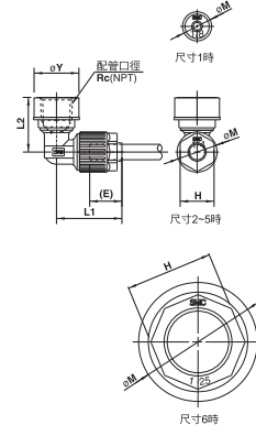
母牙L型彎頭：LQ1L-F
