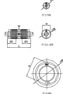
母牙接頭：LQ2H-F
