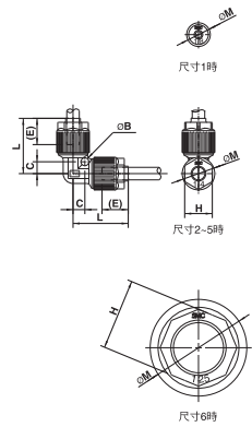
面板安裝連接頭：LQ1P
