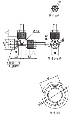
母牙3通接頭：LQ1R-F
